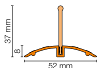
SHOWERPROFILE-WSK + -WSL
