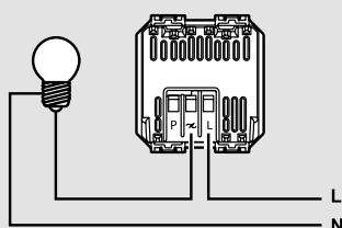
Conexión individual
