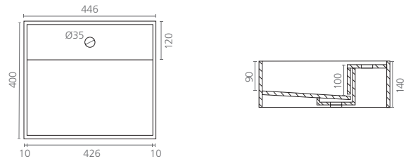
Lavabos de posar Egeo Pivsolid Egeo model sit-on washbasins Vasques à poser modèle Egeo
