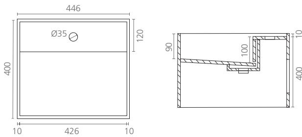
Lavabo de posar o suspendido. Instalación a pared Free-standing or wall-hung washbasin. Wall installation Lavabo à poser ou à suspendre. Installation murale
