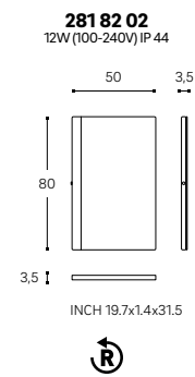
◆ LATERAL LED LIGHT MIRROR ESPEJO CON ILUMINACIÓN LED LATERAL
