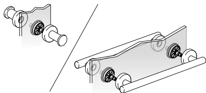
GLASS SHOWER ENCLOSURE HOLDER FOR HOOK / HOOK SOPORTE MAMPARA PARA COLGADOR / COLGADOR GLASS 6/8MM / VIDRIO 6/8MM
