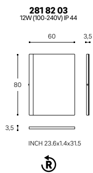
◆ LATERAL LED LIGHT MIRROR ESPEJO CON ILUMINACIÓN LED LATERAL
