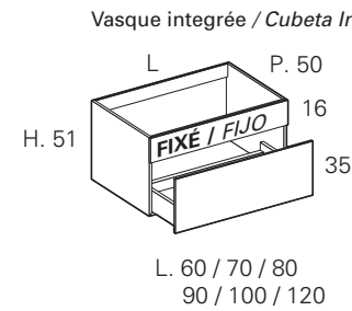
Bases lavabos suspendues H.51 Bases lavabos suspendidas H.51
