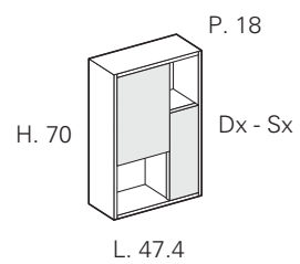
Éléments ouverts mixtes H. 70 Elementos abiertos mixtos H. 70
