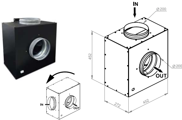
V.2450 ECO Tipo / Type 2
