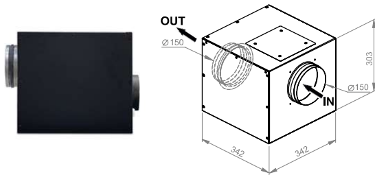
V.2450 ECO Tipo / Type 2
