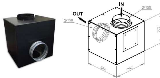
V.3000 N ECO Tipo / Type 2
