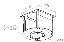
Soporte falso techo regulación de 150 a 240 mm. en rotación (incluido) False Ceiling Support adjustable from 150 to 240 mm. (included)
