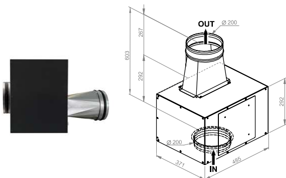
V.2600 ECO Tipo / Type 1
