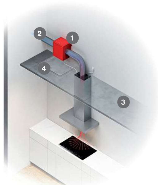
4 Registro acceso al motor Motor access panel
