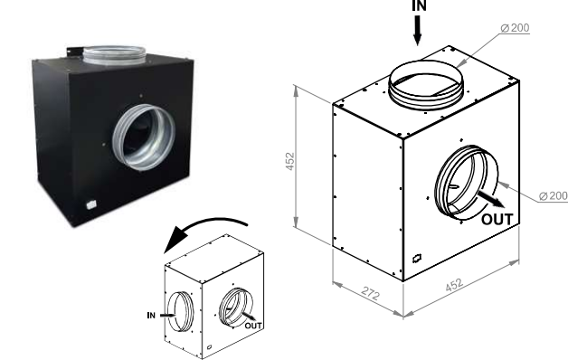
V.3000 N ECO Tipo / Type 2
