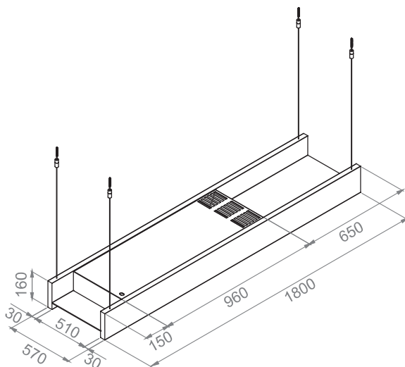
Campana totalmente personalizable tanto en color como en la medida del frontal Fully customizable Cooker Hood in both color and in the size of the front
