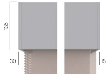
Sistema a cadena Rafter L Eje 44 • Doble cortina
