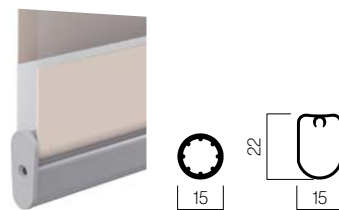
Terminal doble (opcional) 030516
