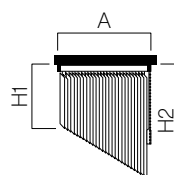
Inclinada. Cabeza horizontal
