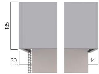
Sistema a cadena Rafter L Eje 65
